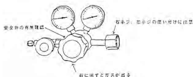
図 9.2 圧力調整器
