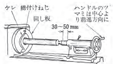
図 4.6 両センタ仕事での留意点
