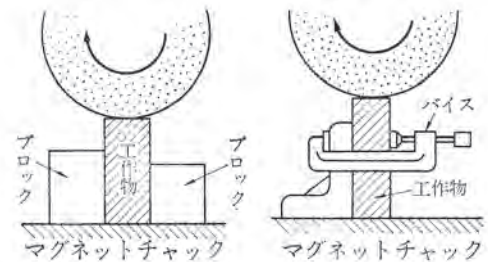
図 4. 7 背の高い工作物の固定方法
