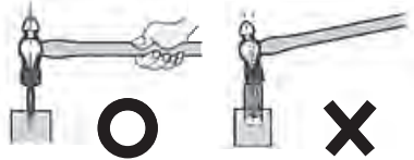
図 4.4 ハンマの打ち方
