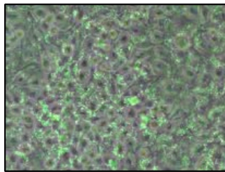
図2. 口腔由来培養細胞と結合した 蛍光ラベル化 S. intermedius
