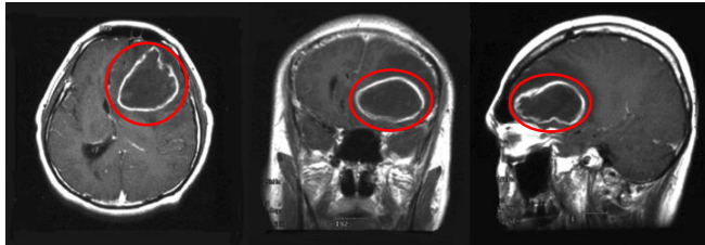
図1. S. intermedius による脳膿瘍
